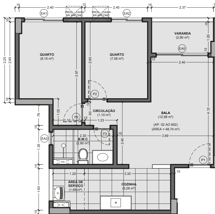
Planta Baixa | apartamentos teminação 02 (Torre 02) | 48,74m 2
