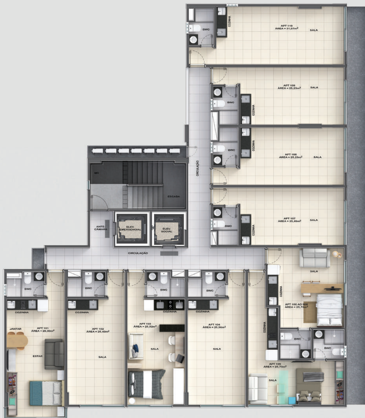
PLANTA HUMANIZADA TIPO 1º
