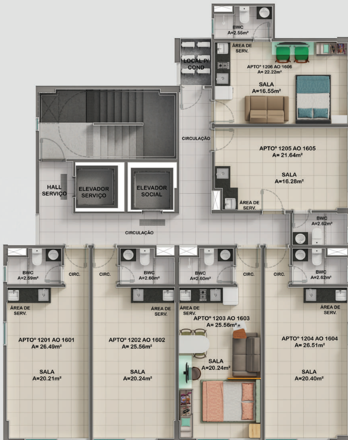
PLANTA HUMANIZADA TIPO 12° AO 16°
