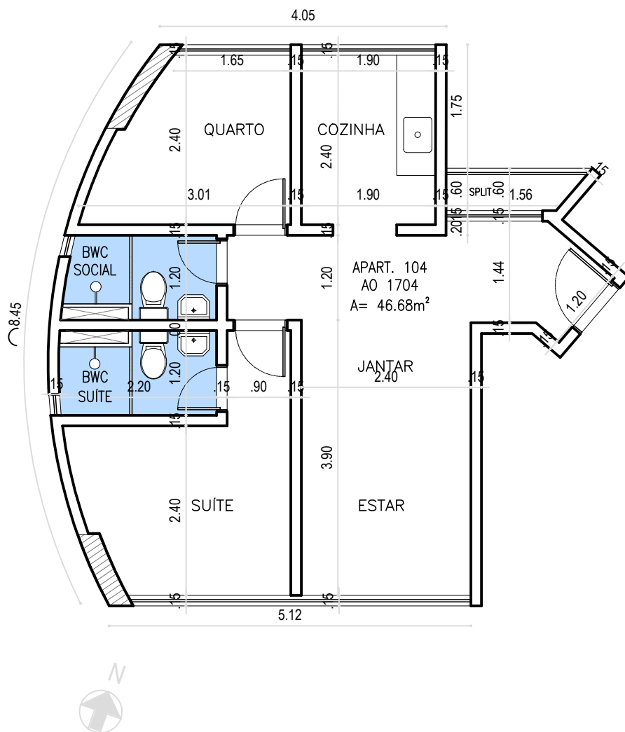
PLANTA BAIXA – APTO. 104 a 1704
