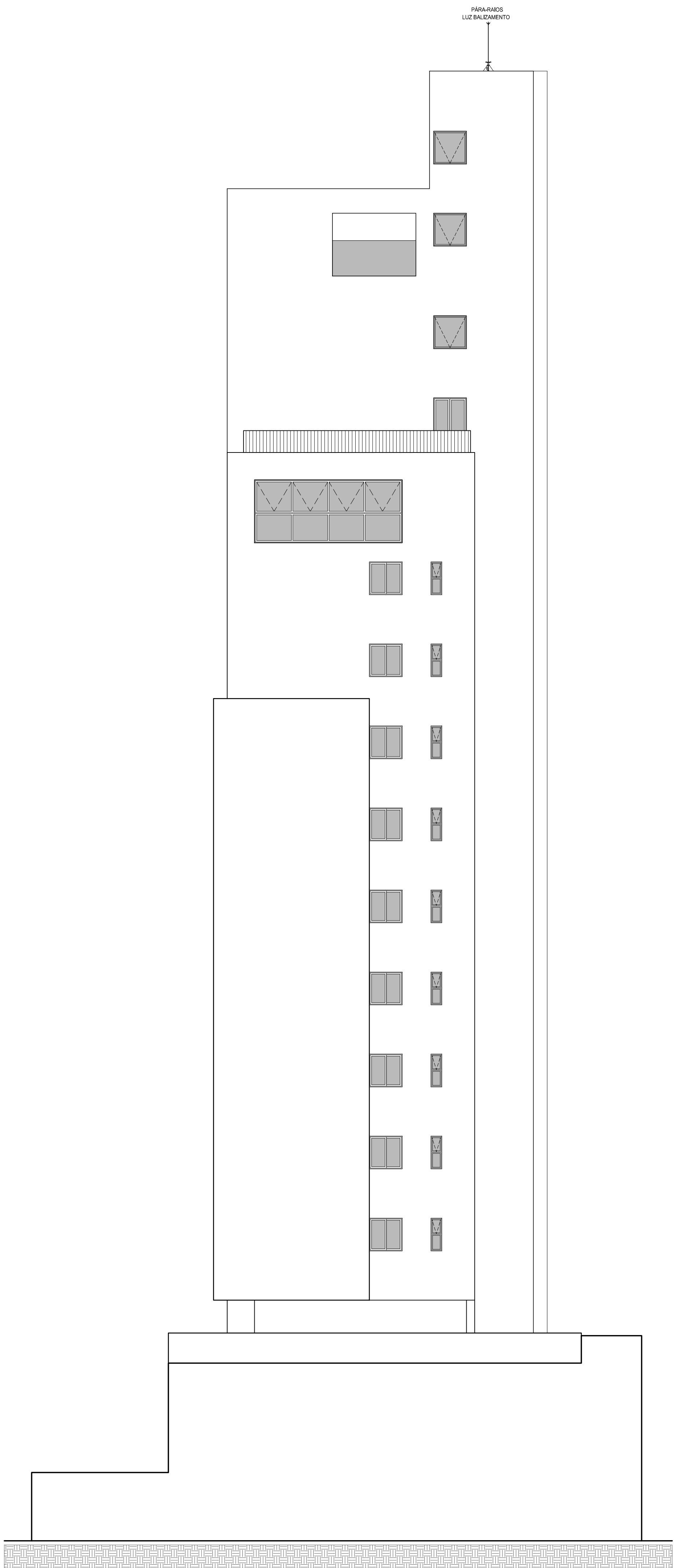
FACHADA - LESTE ESCALA 1/100
